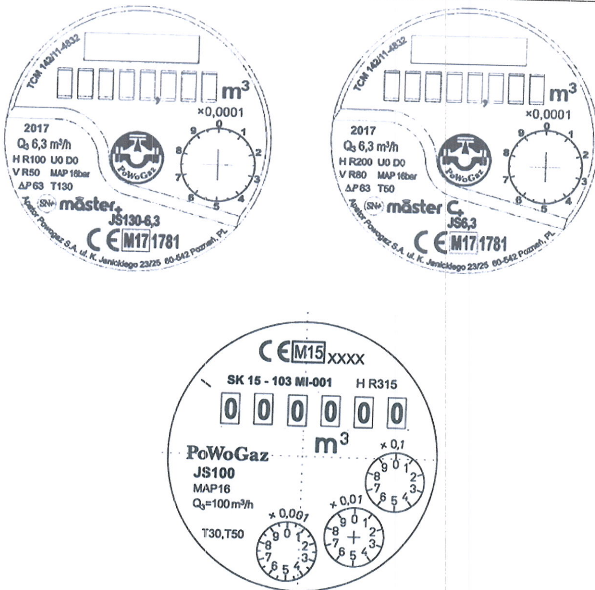
Рисунок 12 – Маркування лічильника
