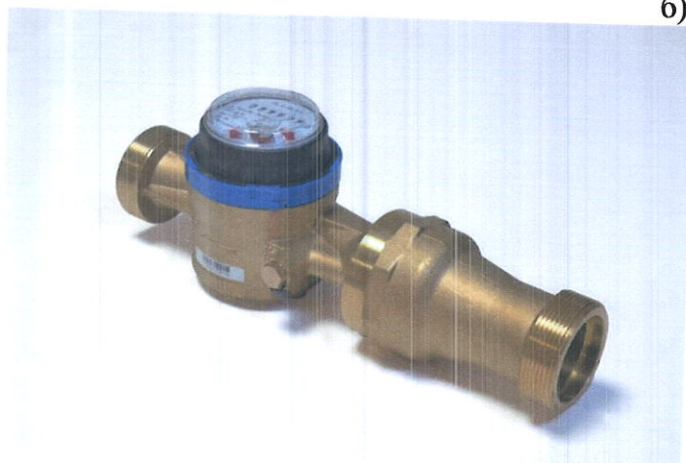
Рисунок 1- Лічильники води модифікації JS... а – загальний вид лічильників номінального діаметру DN15 та DN20; б – загальний вид лічильників номінального діаметру DN15 та DN20 з встановленим імпульсним перетворювачем в – загальний вид лічильника номінального діаметру від DN25 до DN40 г – загальний вид лічильника номінального діаметру від DN25 до DN40 з встановленим імпульсним перетворювачем)
