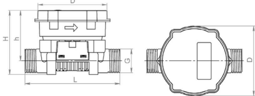
Рисунок 2.1 – Габаритні розміри
