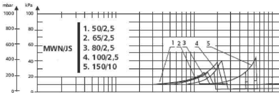
Рис.2 Графік пропускної здатності
