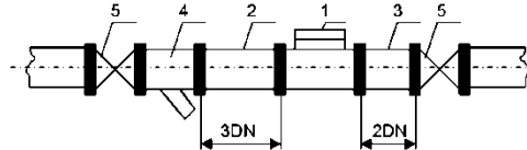
Рис.3 Рекомендована схема встановлення лічильника
